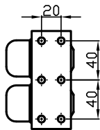
Bohrbild
