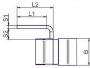
Anschlusschiene, 90° abgewinkelt
