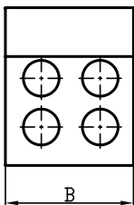
Bolzenbausteine montiert auf E-Cu-Platte
