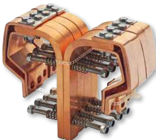
Montagefertige Ersatzkontaktelemente
