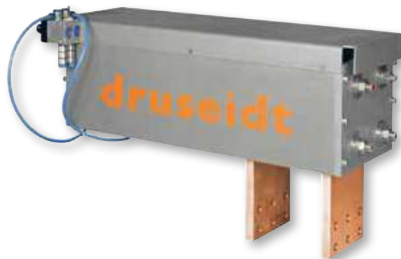
Trennschalter, 1-polig 4000 A
