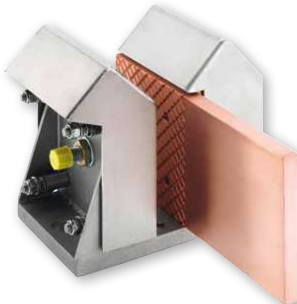
Standardausführung mit gerader Anschlussschiene
