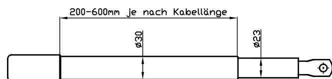
Sonderausführung mit verschweißtem Doppelschlauch
